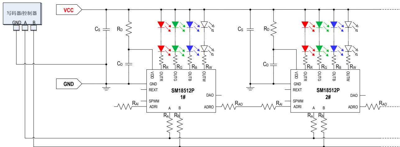
SM18512P 典型应用电路参数包含电源输入电压 VCC, 限流电阻 R_D , 系统电源滤波电容 C_S 和 R/G/B/W LED 分压电阻 R_R 、 R_G 、 R_B 、 R_W , 地址信号输入保护电阻 R_{AI} 以及地址信号输出保护电阻 R_{AO} , A/B 总线信号串接电阻 R_A 和 R_B 。
